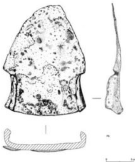
Fig. 28. Casarsa della Delizia, vomere "a lama di vanga" F9 (Disegno L. Blesin, scala 1:2).
