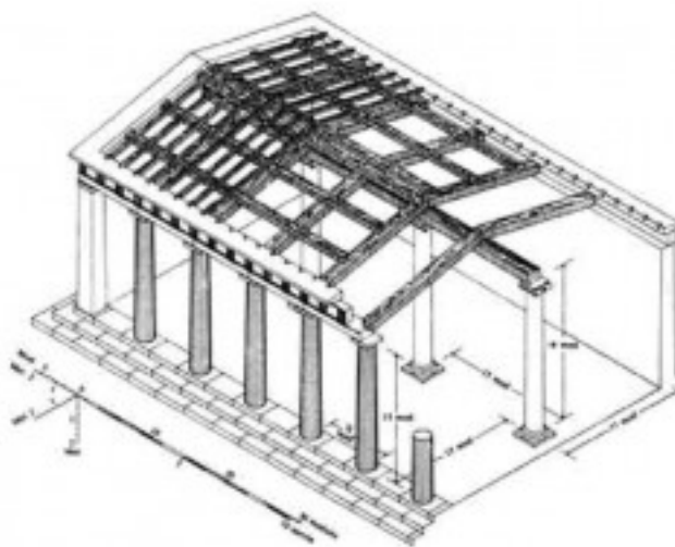
Fig. 6 - Urbis Salvia: ipotesi ricostruttive di una porticus duplex (da COULTON 1976).
