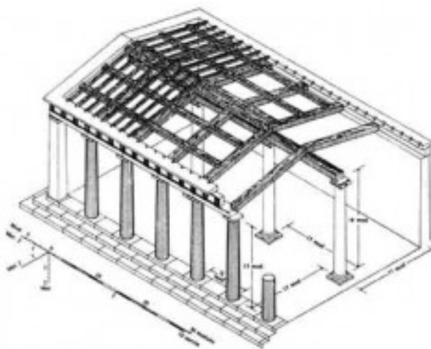
Fig. 6 - Urbis Salvia: ipotesi ricostruttive di una porticus duplex (da COULTON 1975).
