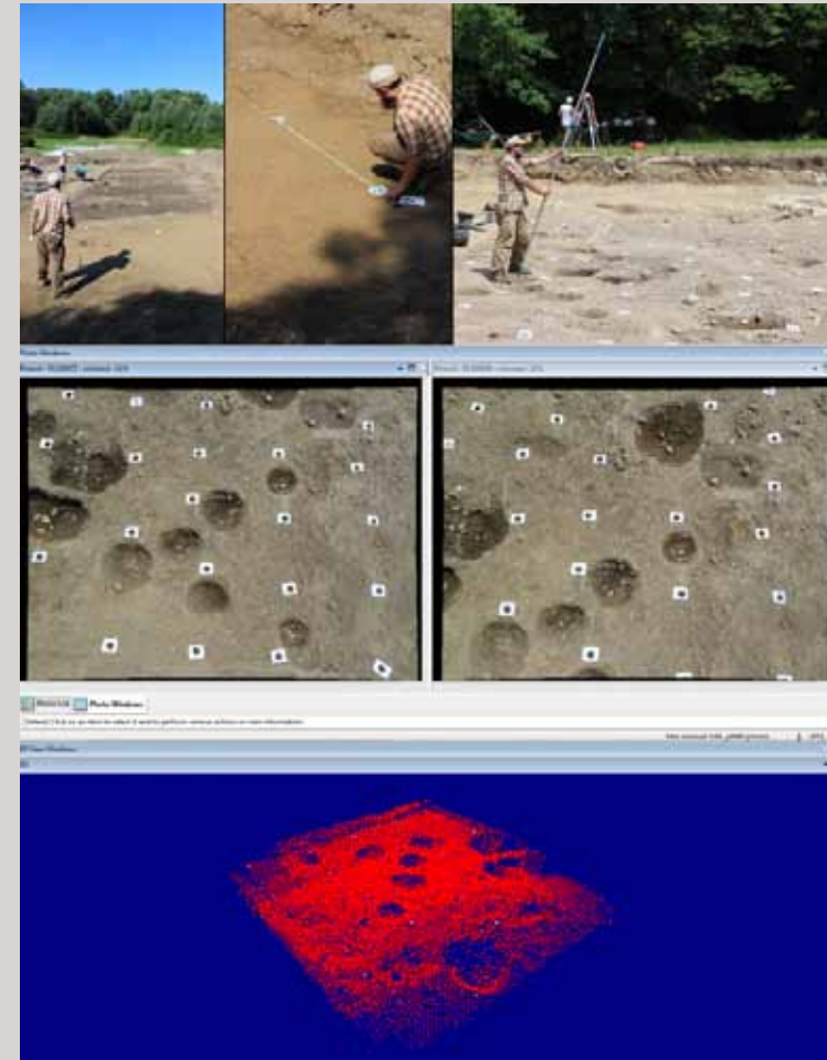
Sequenza operativa per il rilievo fotogrammetrico 3D, dallo strato al modello digitale del terreno.
