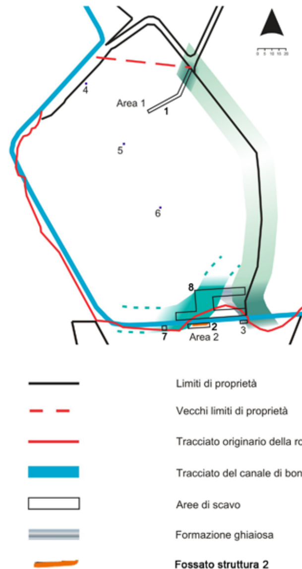
Fig. 21. Rividischia 1998-2000. Planimetria generale degli scavi e ricostruzione delle strutture idrauliche circostanti il castelliere.
